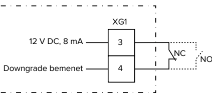
12. Ábra: Elvi kapcsolási rajz: külső kapcsolóérintkező csatlakoztatása (alapbeállítás: NC)
