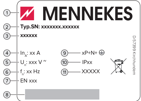
Afb. 1: Typeplaatje (monster)
