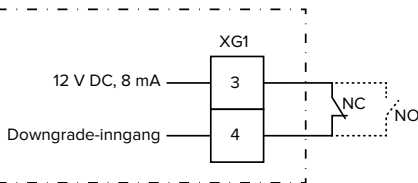
Fig. 12: Prinsipielt koblingsskjema: tilkobling av en ekstern bryterkontakt (standardinnstilling: NC)
