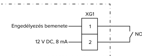
13. Ábra: Elvi kapcsolási rajz: külső kapcsolóérintkező csatlakoztatása
